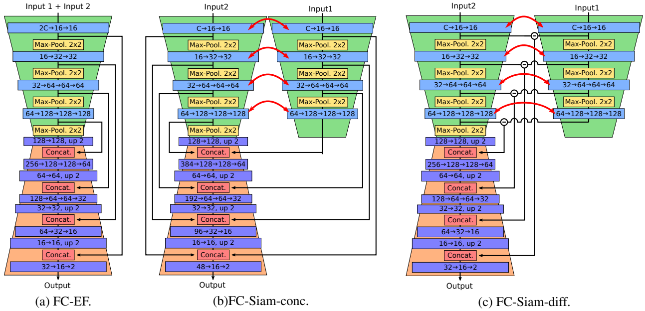
FIGURE 2 – Schémas des trois architectures FCNN proposées pour la détection de changements. Couleur des blocs : le bleu est la convolution, le jaune le max pooling , le rouge est la concaténation, le violet est la convolution transposée. Les flèches rouges illustrent les poids partagés entre les composants siamoises du réseau.
