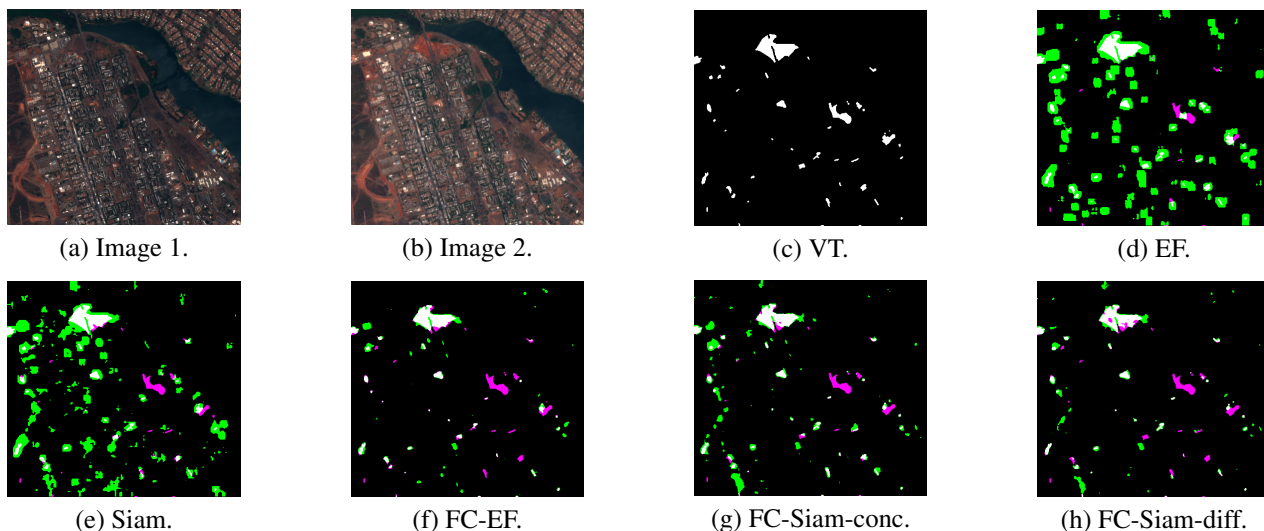
FIGURE 4 – Résultats de test sur brasil de la base OS2UC, avec les 13 canaux de couleur. Dans les images (d), (e), (f), (g) et (h), le blanc correspond au vrai positif, le noir au vrai négatif, les faux positifs sont en vert et les faux négatifs en magenta.
